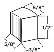
Cubelet Dimensions
